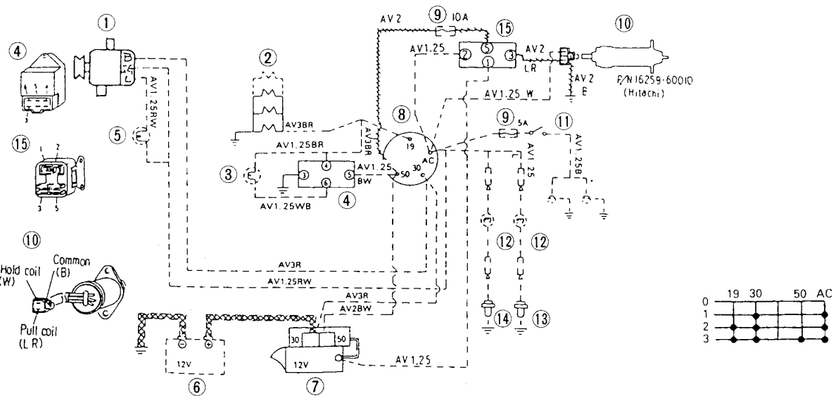
Połączenie wewnętrzne stacyjki
