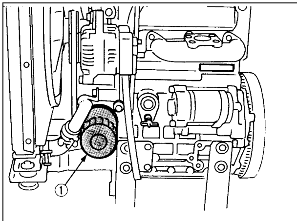
(1) Wkład filtra oleju Wykręcić za pomocą klucza do filtrów (Dokręcić ręcznie)
